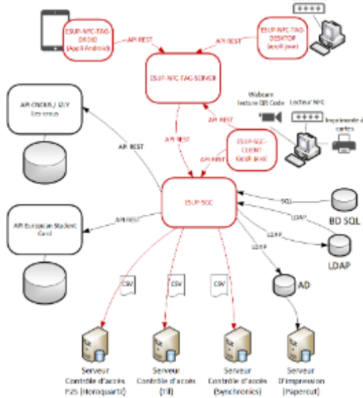
Architecture logicielle
