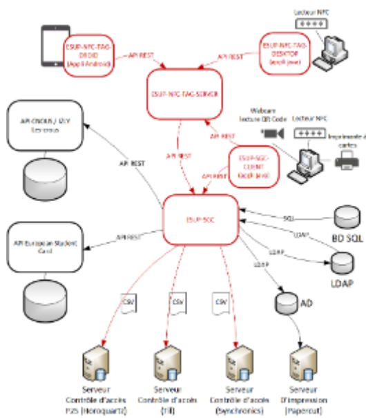
Architecture logicielle
